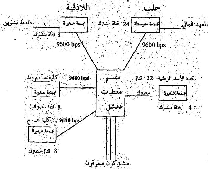
شكل 9-أ البنية العامة لشبكة Syrialink
